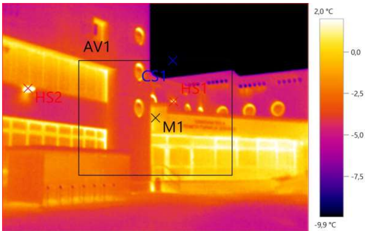
Slika 1: Termo slika – OŠ Tone Čufar
