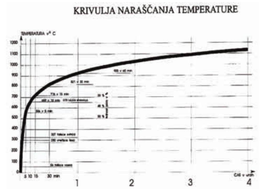
Faze razvoja požara – požarna krivulja
